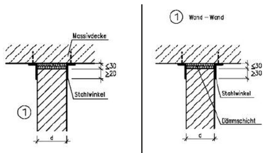
Bild 4: Anschlüsse nach DIN 4102-4
